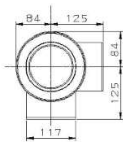
L (2口)
