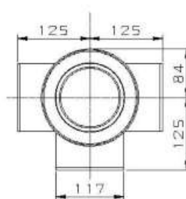
T (3口)
