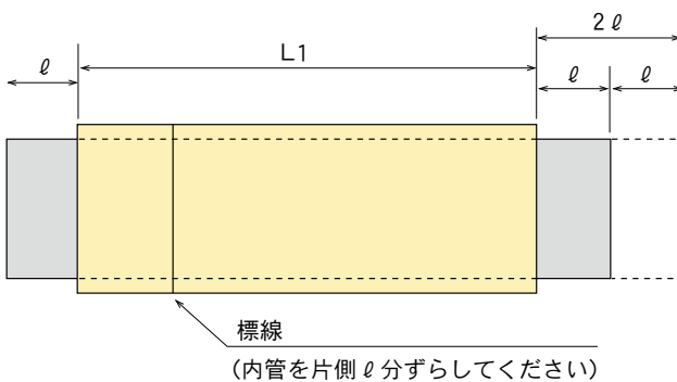
塩ビ内管の挿入代 単位 (mm)
