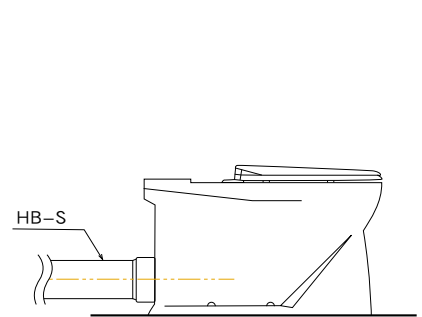
③ HB-S 接続例
