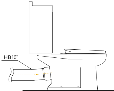
② HB10° 接続例
