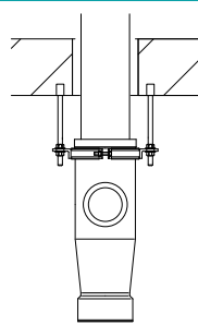
天井吊り下げ固定
