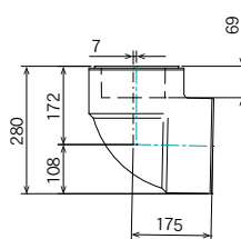
XJ-B CE (VUH) 150×125
