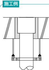
スラブ下固定タイプ
