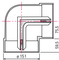
■ 水平90°エルボ VM125LH
