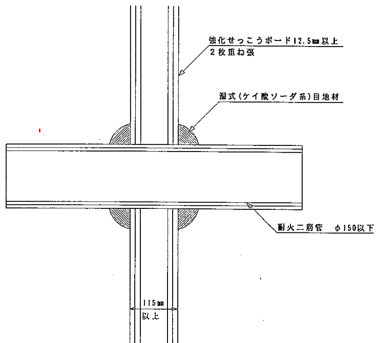
給排気管（耐火二層管）の防火区画（中空壁）貫通部措置工法
