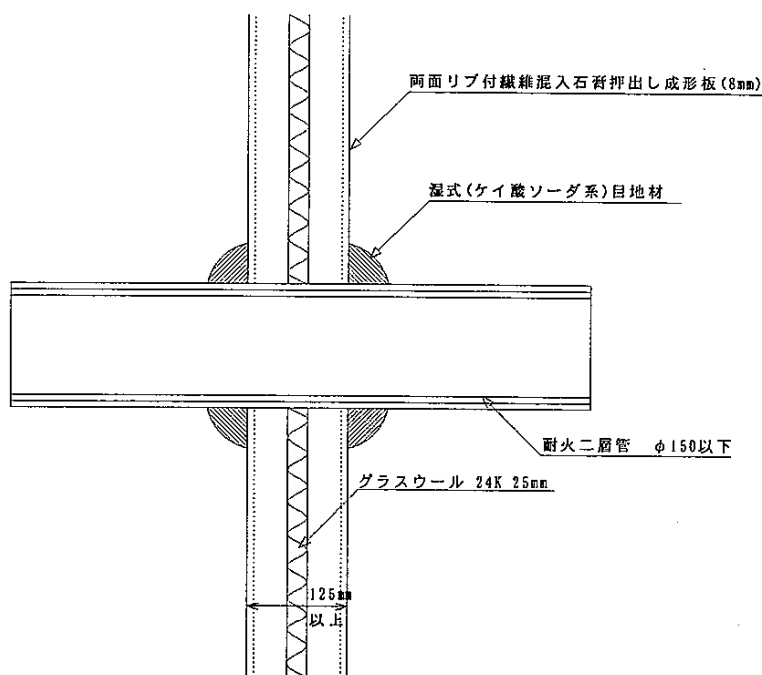
給排気管（耐火二層管）の防火区画（中空パネル壁）貫通部措置工法
