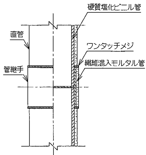
標準仕様の断面詳細①
