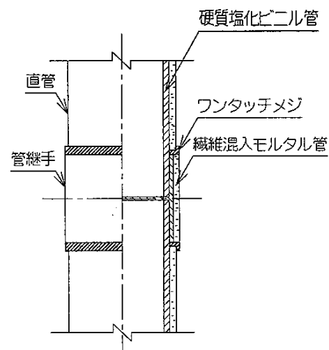
標準仕様の断面詳細③
