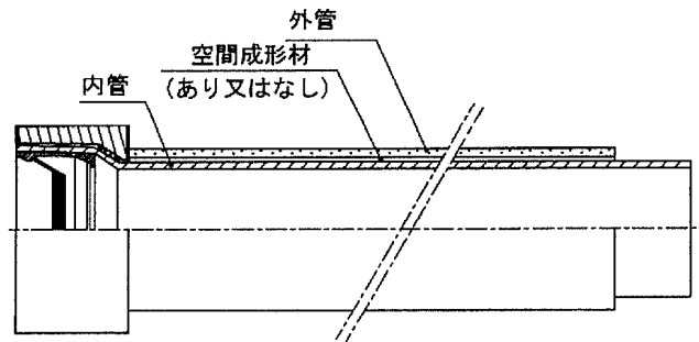
図-3 受け口耐火二層管
