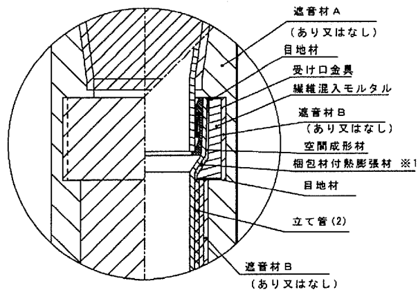
※1 梱包材付熱膨張材を使用しない場合は、横枝管を耐火二層管とする 図-2 受口部詳細
