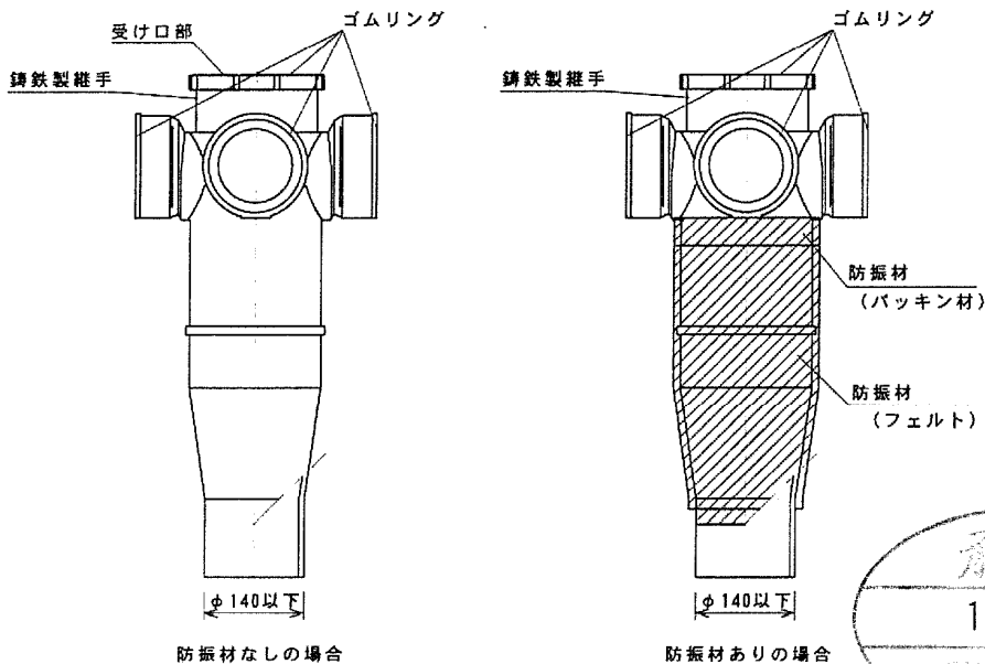
図-6 鋳鉄製継手の例図
