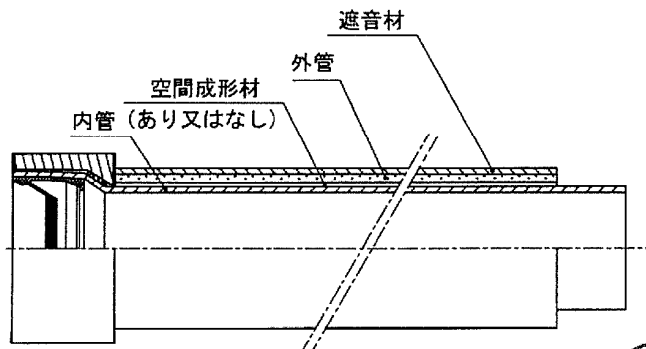
図-4 遮音型受け口耐火二層管
