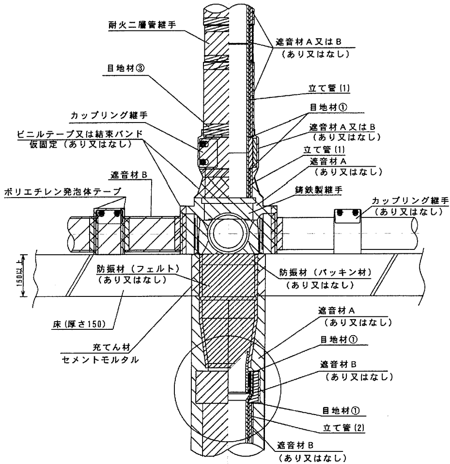
図-1 防振材あり配管例
