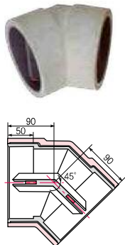
■ 水平45°エルボ FPVM125 45LHW
