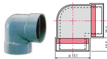
■ 垂直90°エルボ VM125LV
