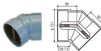
■ 水平45°エルボ VM125・45L
