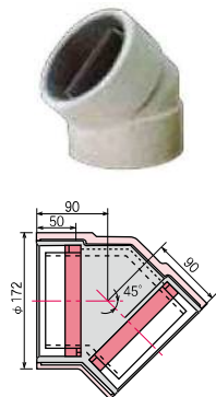
■ 垂直45°エルボ FPVM125 45LVW
