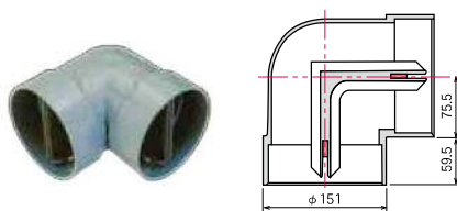
■ 水平90°エルボ VM125LH
