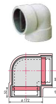
■ 垂直90°エルボ FPVM125 LVW
